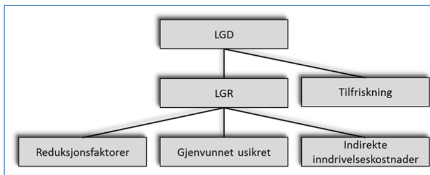
Figur 7 - Oppbygging, LGD-modellen
